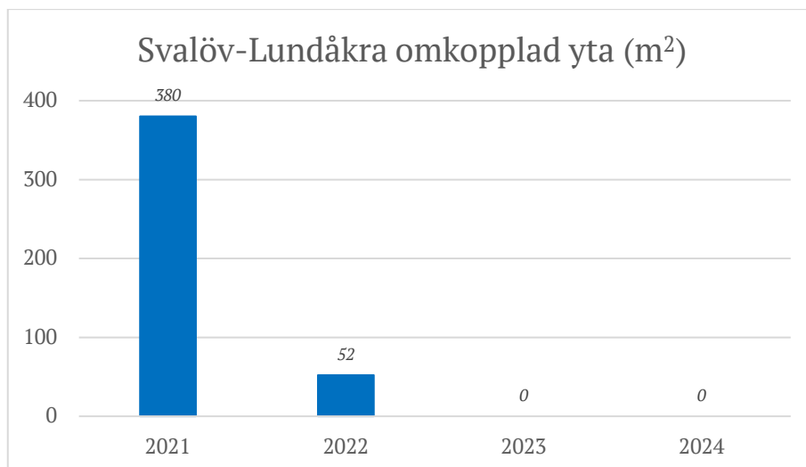
Figur 5. Översikt över bortkopplade hårdgjorda ytor i m² åren 2021–2024.
