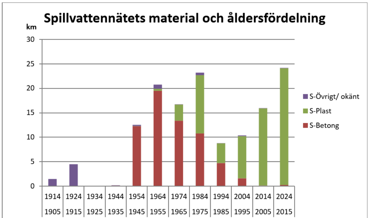
Figur 6. Spillvattennätets nuvarande material- och åldersfördelning från Svalöv Strategisk Reinvesteringsplan för VA-ledningsnätet 2024.
