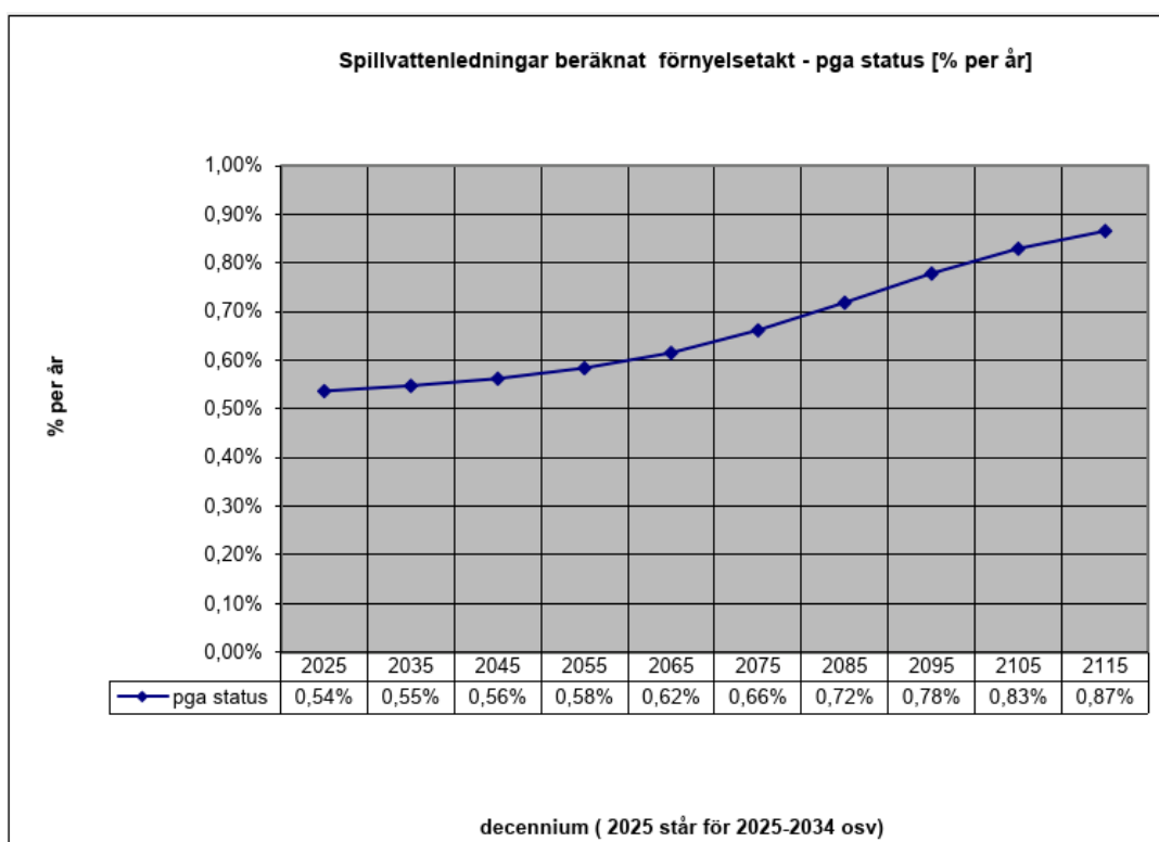
Figur 7. Svalövs kommun - reinvesteringstakt för spillvattennätet de närmsta 100 åren (procent av befintlig ledningslängd).
