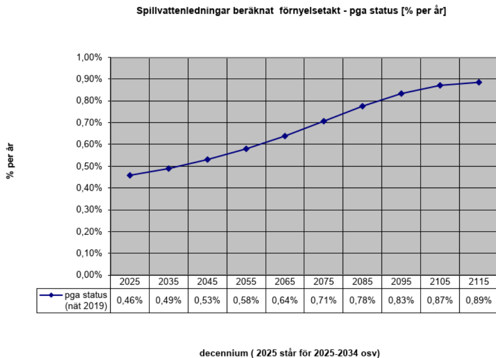
Figur 14. Åstorp - reinvesteringstakt för spillvattennätet de närmsta 100 åren (procent av befintlig ledningslängd)
