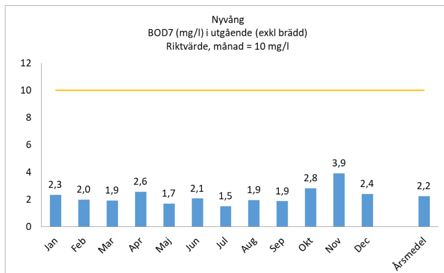
Figur 7. Sammanställning av utgående BOD 7 halt och villkorsefterlevnad, per månad och år.
