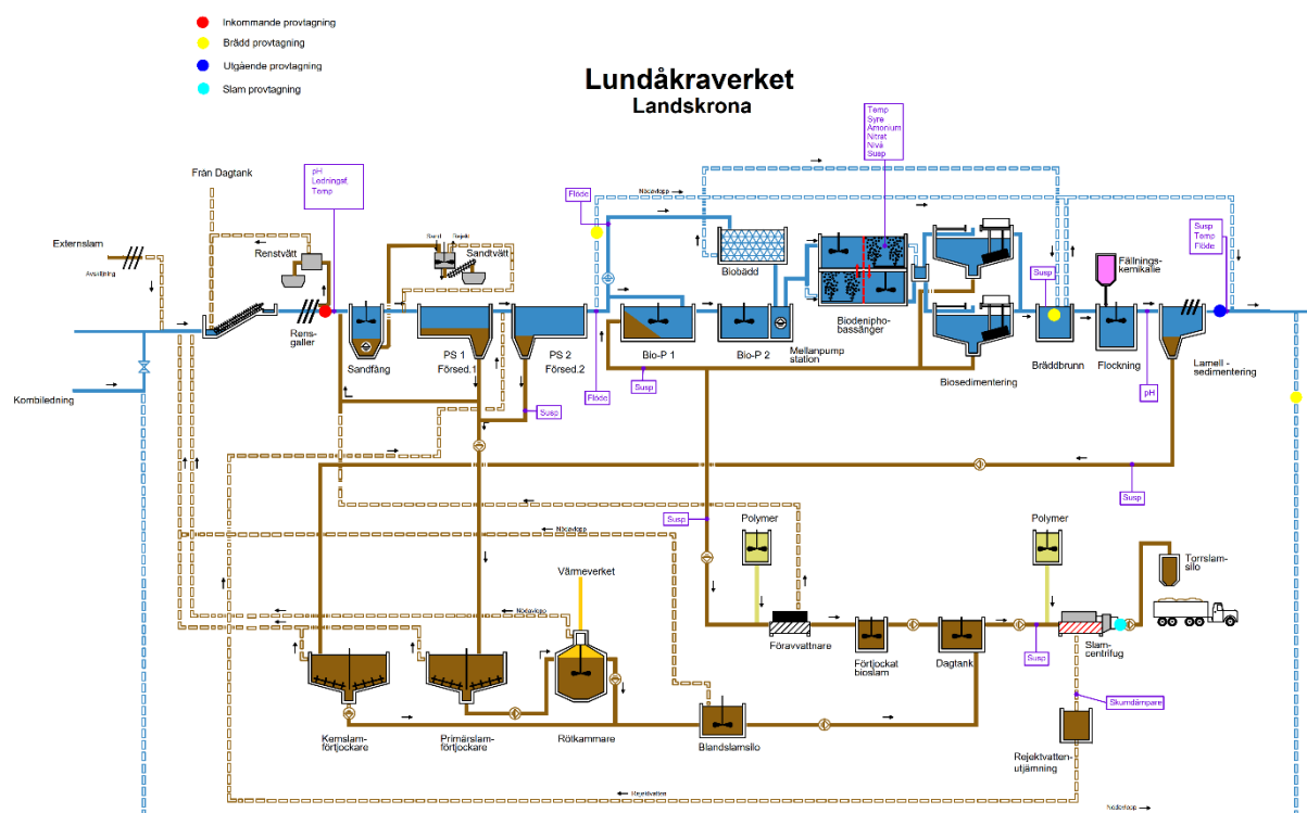
Figur 6. Processchema Lundåkraverket.
