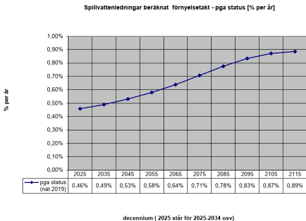
Figur 11. Åstorp - reinvesteringstakt för spillvattennätet de närmsta 100 åren (procent av befintlig ledningslängd)
