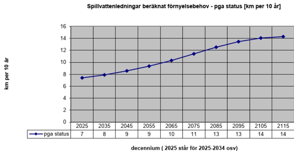
Figur 12. Åstorp - Reinvesteringstakt för spillvattennätet i km ledningslängd per decennium de närmsta 100 åren
