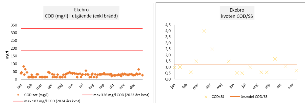
Figur 11. Utgående totalt COD, beräknad COD-gräns och COD/SS-kvot under 2024.
