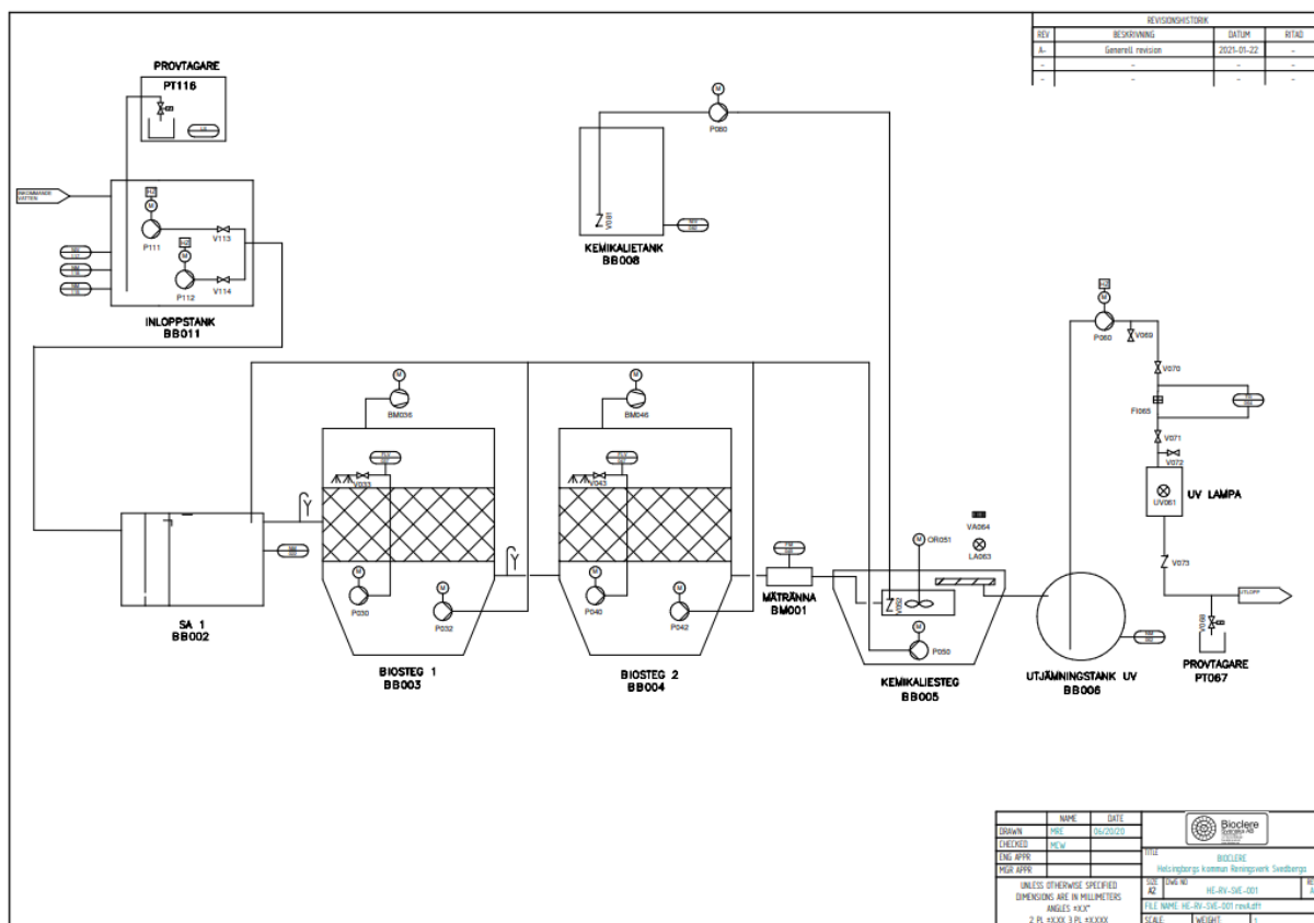
Figur 4. Visar ett processchema över reningsverket.
