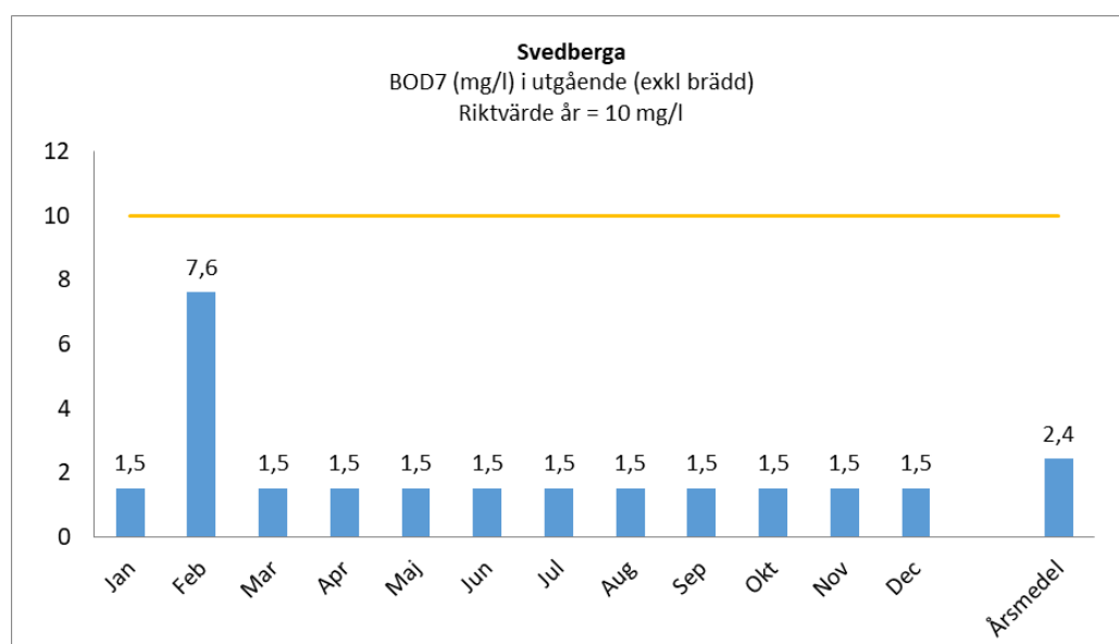
Figur 5. Visar utgående BOD i mg/l för alla månader under året, samt årsmedelvärdet.
