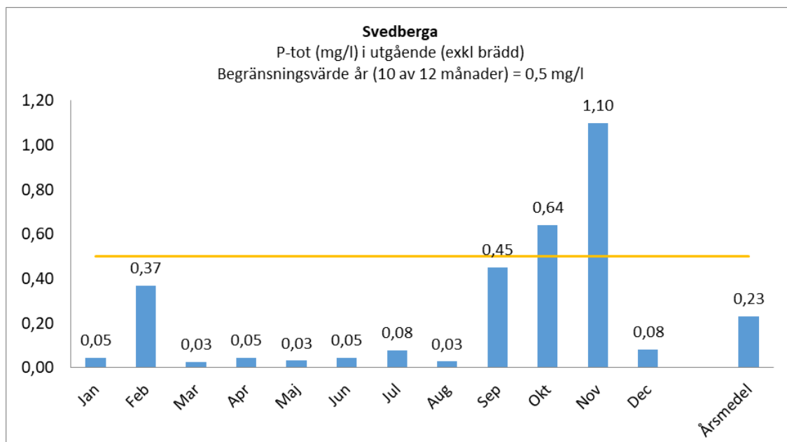
Figur 6. Visar utgående totalfosfor i mg/l för alla månader under året, samt årsmedelvärdet för samtliga månader vilket låg på 0,23 mg/l. För 10 av 12 månader låg årsmedelvärdet på 0,18 mg/l.
