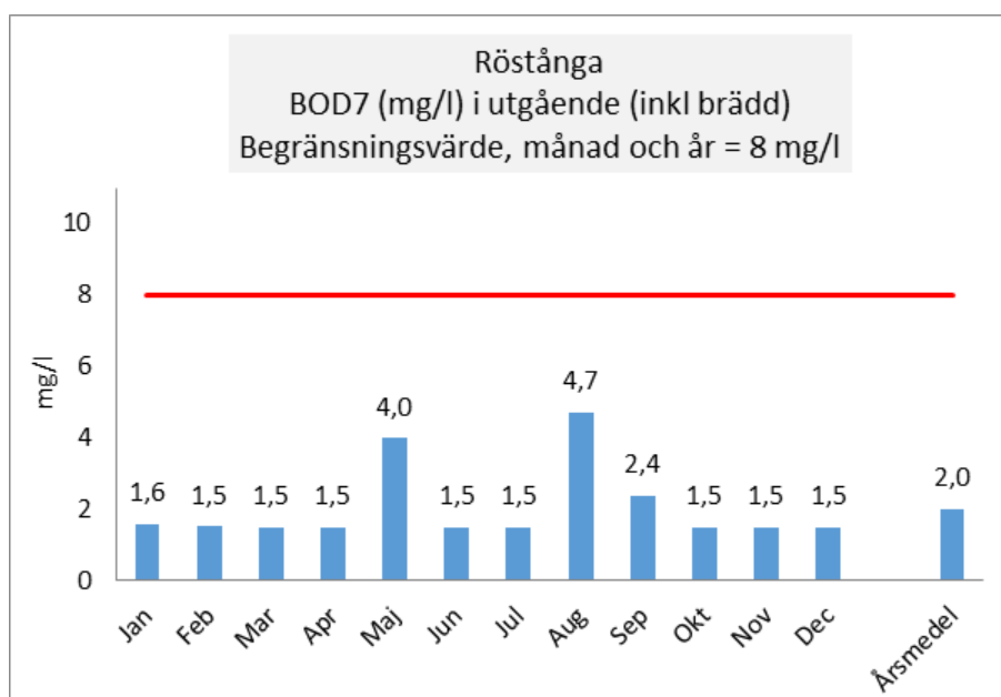
Figur 7. Utgående halt BOD 7 från Röstånga avloppsreningsverk.
