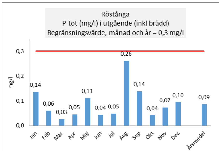
Figur 8. Utgående halt totalfosfor från Röstånga avloppsreningsverk.
