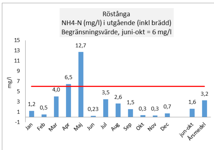
Figur 9. Utgående halt ammoniumkväve från Röstånga avloppsreningsverk.
