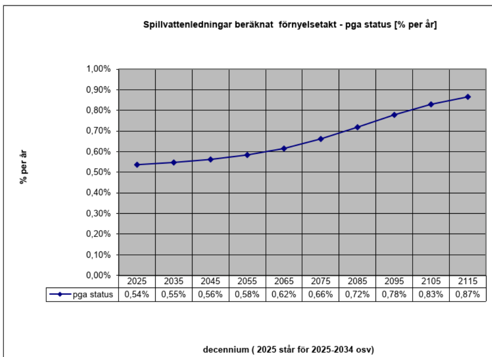
Figur 12. Svalöv - reinvesteringstakt för spillvattennätet de närmsta 100 åren (procent av befintlig ledningslängd).
