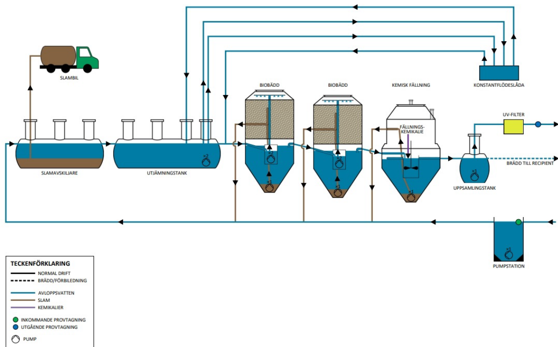
Figur 4. Visar ett översiktligt processchema över verket.
