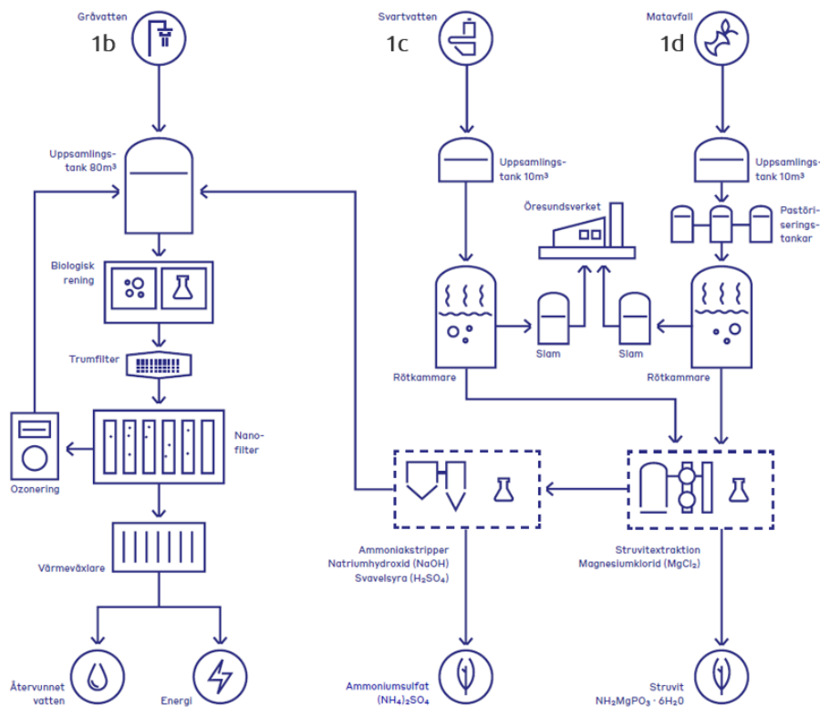
Figur 8. Processschema över RecoLab. Schemat visar provtagningspunkter där provpunkt 1b är för inkommande gråvatten, provpunkt 1c är för inkommande svartvatten och provpunkt 1d är för inkommande matavfall.
