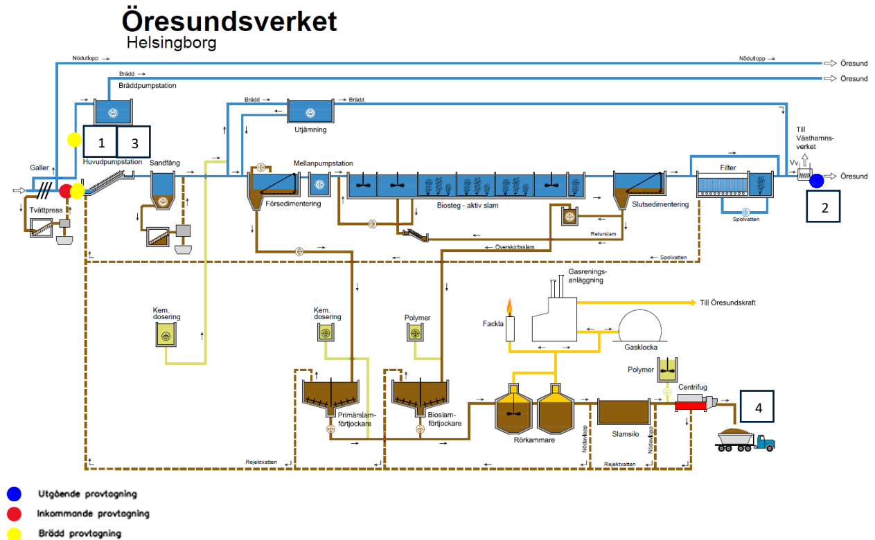
Figur 7. Processschema över Öresundsverket (exklusive RecoLab). Schemat visar provtagningspunkter där provpunkt 1 är för inkommande avloppsvatten, provpunkt 2 är för utgående avloppsvatten och provpunkt 3 är provpunkt för bräddat avloppsvatten, 4 avvattning.
