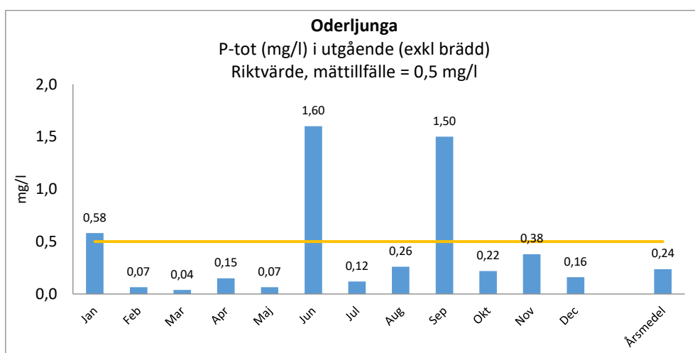
Figur 6. Utgående halt P-tot från Oderljunga avloppsreningsverk
