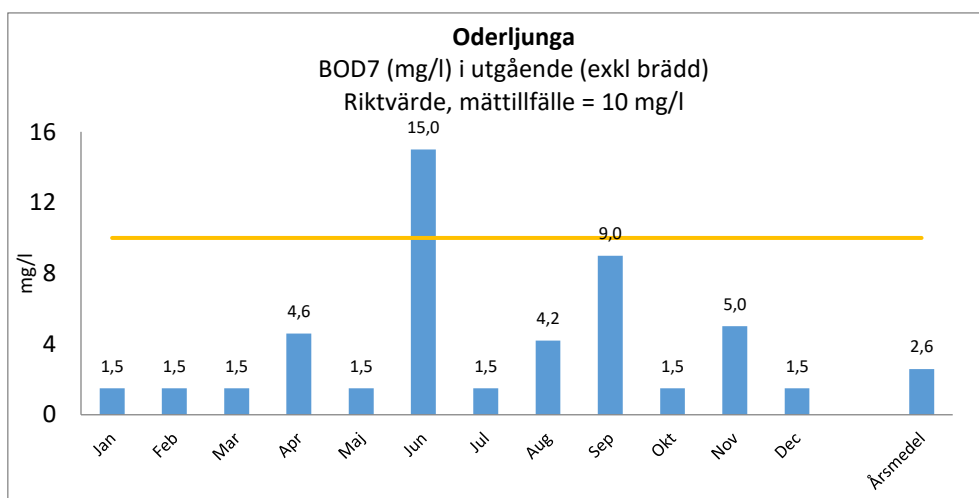
Figur 5. Utgående halt BOD 7 från Oderljunga avloppsreningsverk
