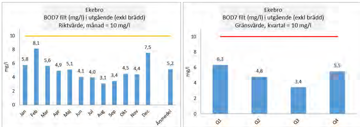
Figur 7. Utgående halt BOD 7 från Ekebro avloppsreningsverk.
