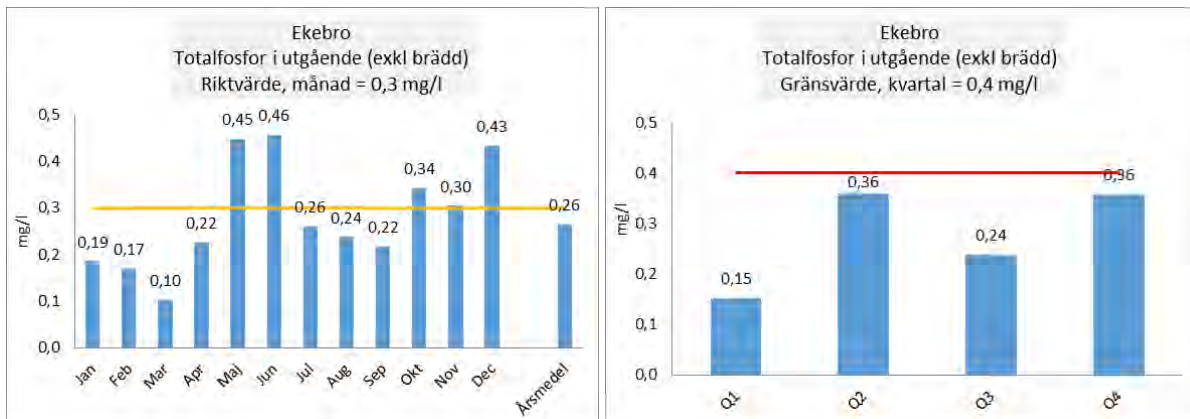
Figur 8. Utgående halt totalfosfor från Ekebro avloppsreningsverk.
