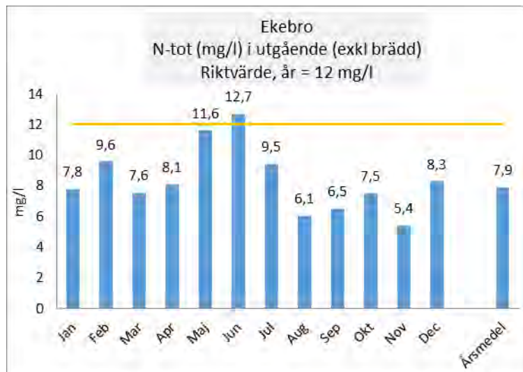
Figur 9. Utgående halt totalkväve från Ekebro avloppsreningsverk.
